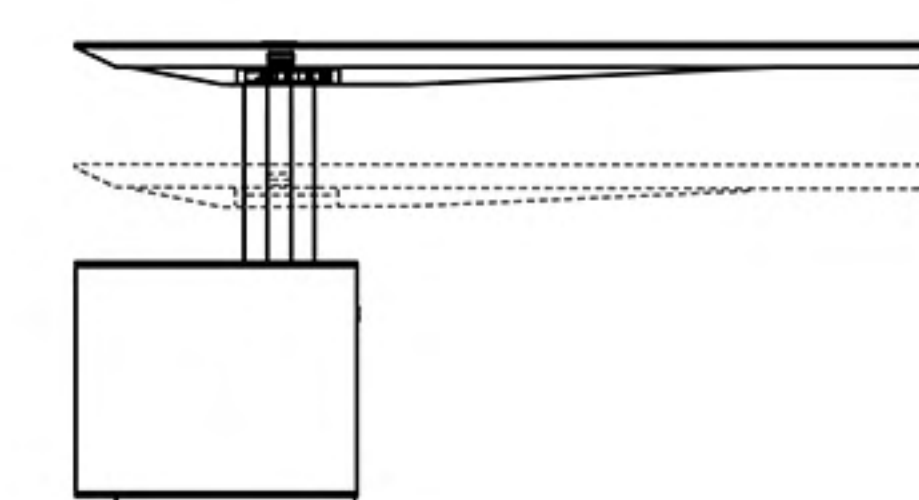
LH-L 2200 / 700 / 750~1175
