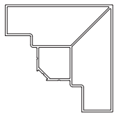
L型柱B 7136#
