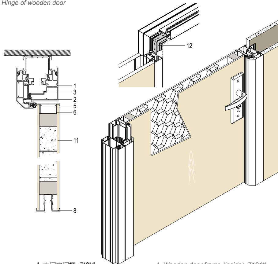
木门门铰 Hinge of wooden door
