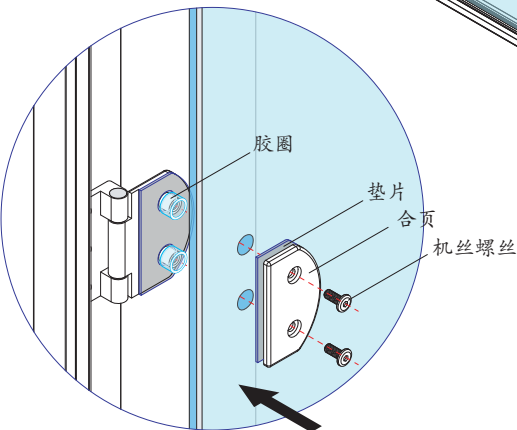
2.将玻璃门对准孔用机丝把门合页锁紧
