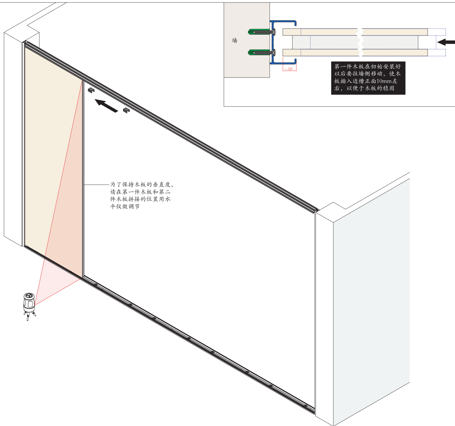
天槽木板固定件
