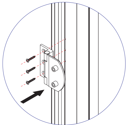
1.将合页用自攻螺丝固定在玻璃门内门框上
