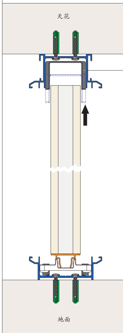
天槽木板固定件
