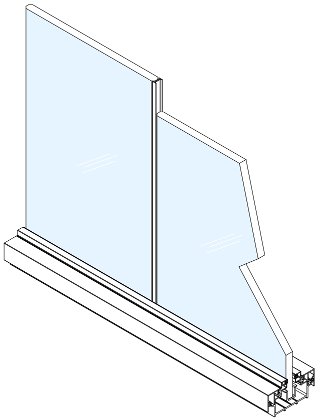
1. 玻璃双边连接条(12mm) FU182-003# 1. Double glass groove FU182-003#
